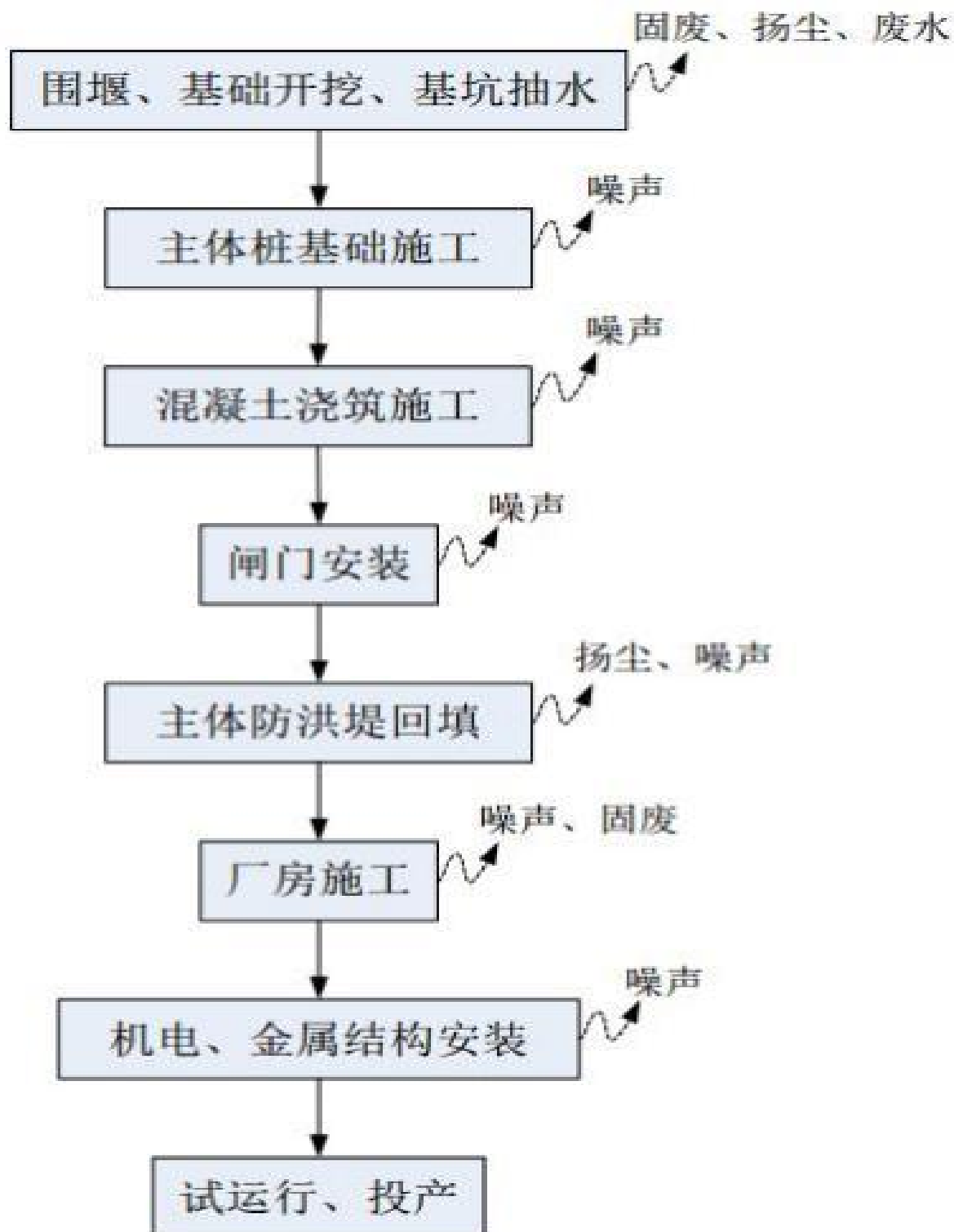
图 3-6 项目建施工工艺流程示意图
